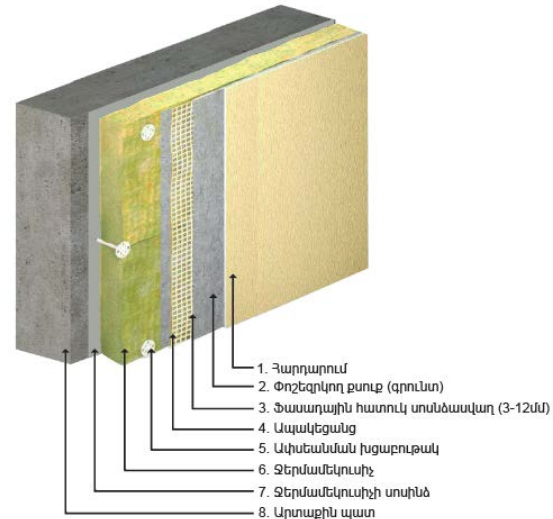
Նկ. 1 Էքստրուդացված պոլիստիրոլի կամ հանքային բամբակի սալերով ջերմամեկուսացում
