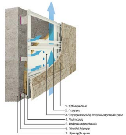
Նկ. 13 Օդափոխվող օդային միջնաշերտով պատի ջերմամեկուսացումը փոփոխականությամբ
